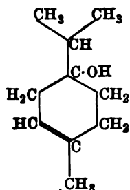
Terpinenol.
